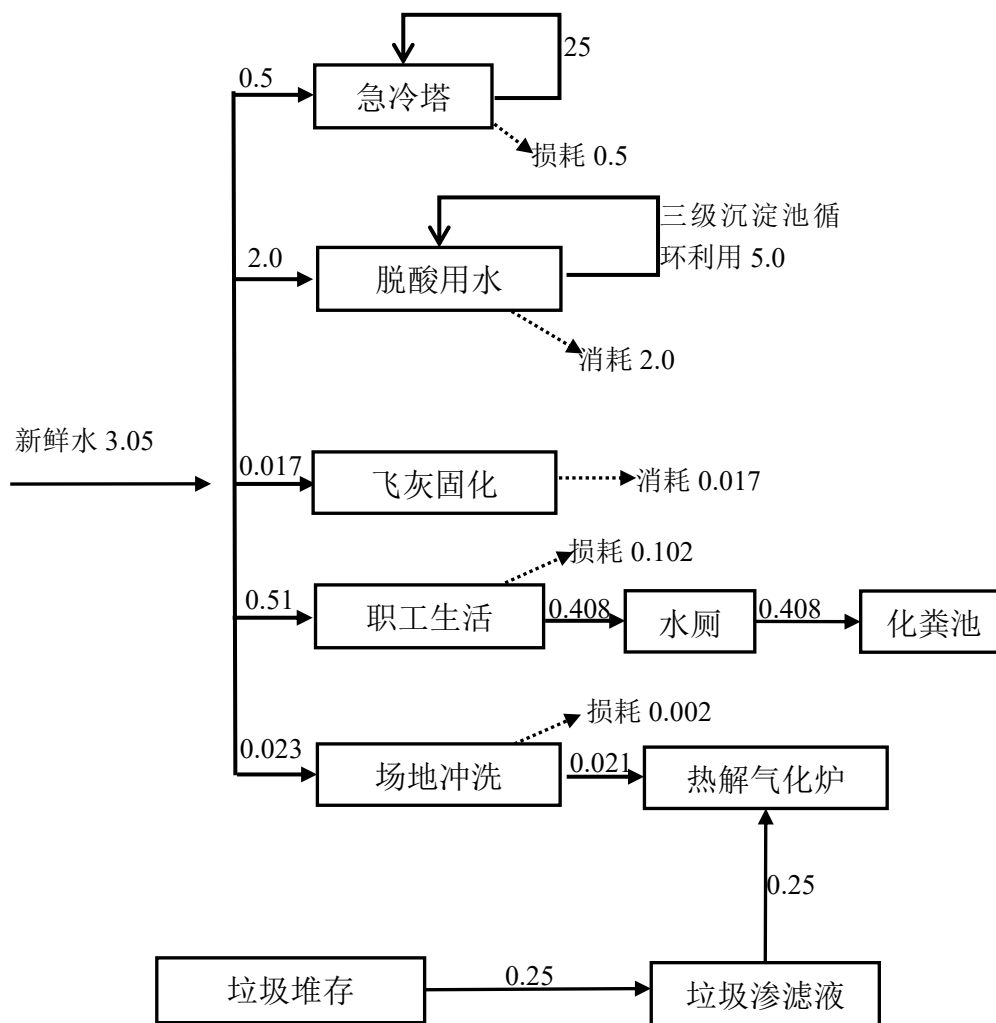
图 3-4 本项目水平衡图 ( \text{m}^3/\text{d} )
