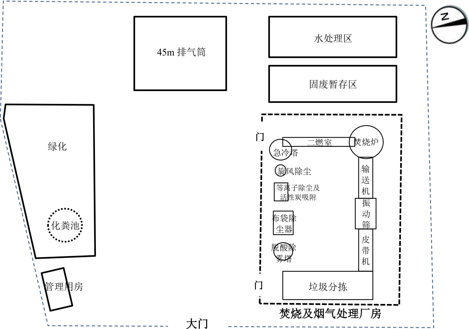
图 3-3 项目平面布置图
